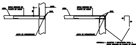
DETALLE ALTERNATIVO SUPLES EN MUROS
